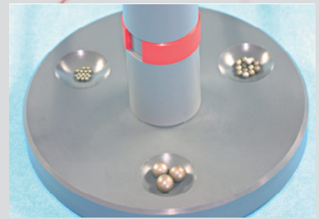
Pied de mesure avec empreintes pour garder les billes de référence en place durant la mesure
